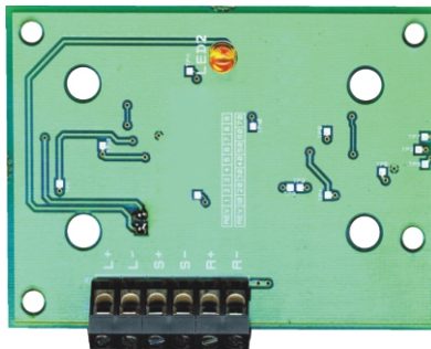
FIG. 3 FC410LI Placca Facia Plate Kurzschlussisolator Vorderseite
